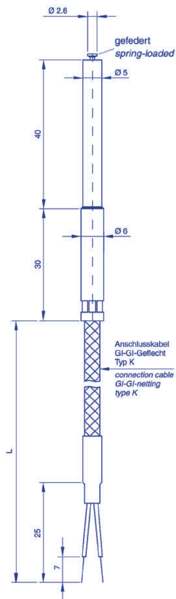
Oberflächentastfühler mit Kabel Surface touch probe with cable
