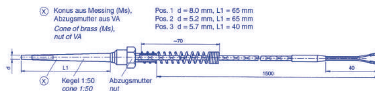
Konischer Einschraubfühler Cone screw-in probe
