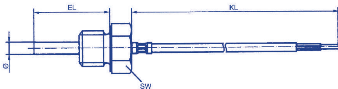
Maßzeichnung Dimensional drawing
