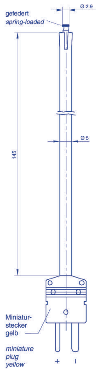
Tastfühler mit Miniaturstecker Touch probe with miniature plug
